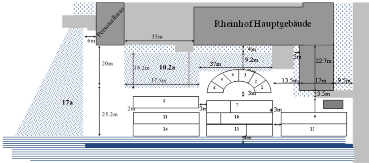
Situationsplan Sortenschaugarten Rheinhof
